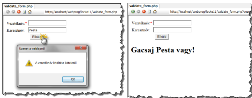
93. ábra Hibaüzenet, és helyes kitöltés után visszakapott oldal
