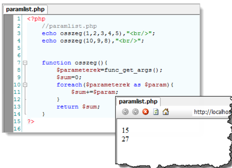
57. ábra Változó számú paraméterek
