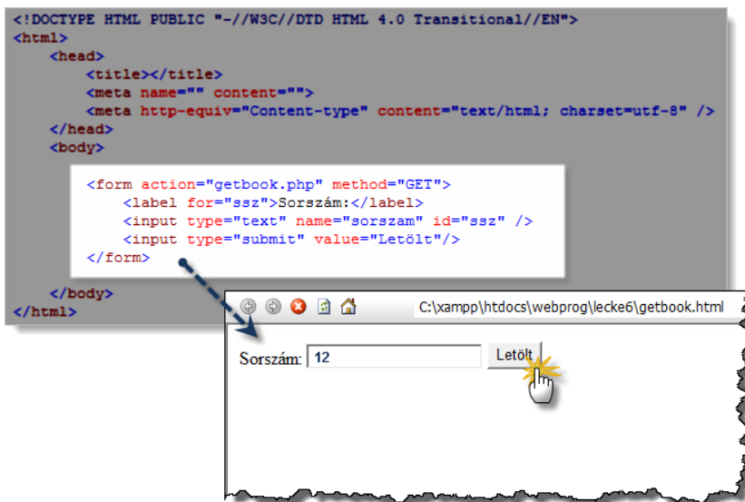
35. ábra HTML-űrlap a böngészőben
