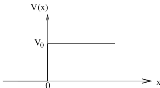
2.27. ábra. Potenciállépcső potenciálja.
