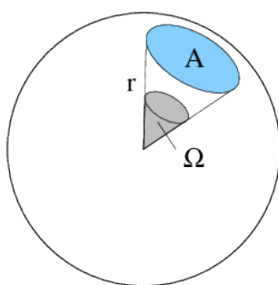
1.4. ábra. A térszög definíciója az ábrának megfelelően \Omega = \frac{A}{r^2} . A teljes térszög \Omega = 4\pi .
