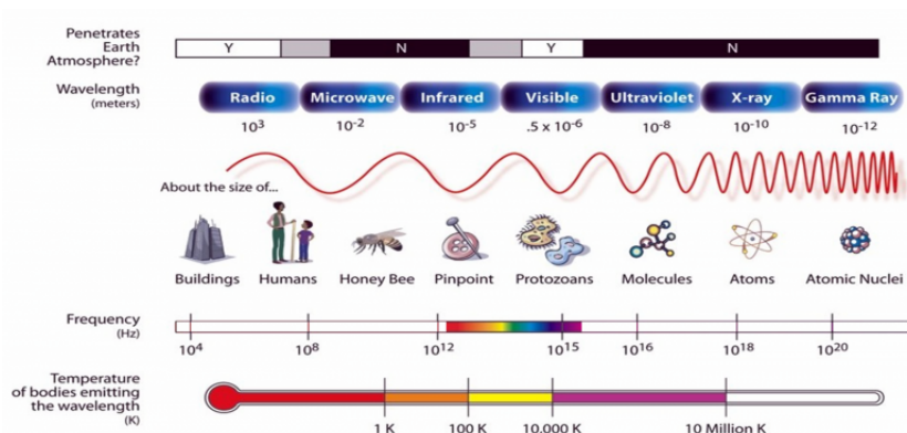
2.1. ábra. Az elektromágneses sugárzás spektruma. mmi.oregonstate.edu
