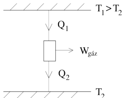
1.33. ábra. Carnot-körfolyamat, mint a hőerőgép modellje. A két hőtartállyal kapcsolatba hozott gép a T_1 hőmérsékleten Q_1 hőt felvesz, a T_2 < T_1 hőmérsékleten Q_2 hőt lead, miközben W^{\text{gáz}} munkát végez. A megfelelő betűk már csak nagyságot jeleznek, előjelük a nyilaknak megfelelő.
