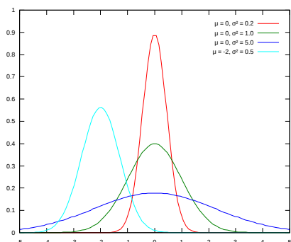
Gauss-féle normál-eloszlás függvények. Haranggörbének is nevezik.
