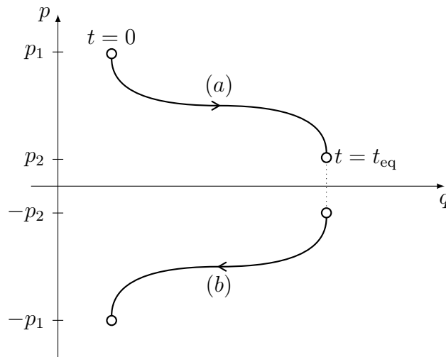
1.3. ábra. Loschmidt-féle reverzibilitási paradoxon: az (a) relaxációs folyamat (b) időtükrözöttjét sosem tapasztaljuk, holott az is megfelel a mikroszkopikus dinamikának
