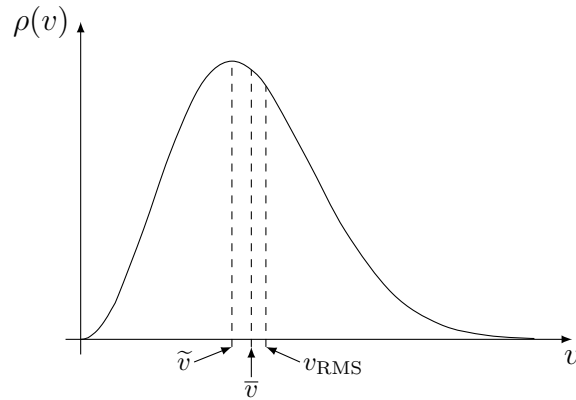
1.19. ábra. A Maxwell-féle sebességeloszlás a \tilde{v} legvalószínűbb, a \bar{v} átlagos és a v_{\text{RMS}} = \sqrt{\overline{v^2}} átlagos négyzetes sebességgel.
