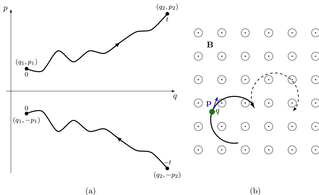
5.1. ábra. (a) Időtükörözött trajektóriák (b) A rendszer paramétereit is transzformálni kell, ellenkező esetben a (q, p) \mapsto (q, -p) , t \mapsto -t transzformáció nem felelne meg az időtükrözésnek, így a tükrözés után a szaggatott pályát követné a részecske
