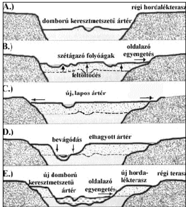
6. ábra A folyó életfolyamatai öt ételben
