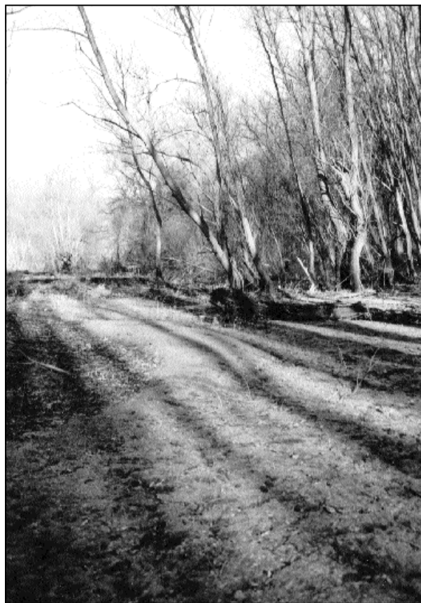
2. ábra A sodorvonalból kiszoruló víz hordalékterítése.
