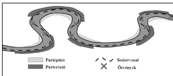
1. ábra Mederváltozások a folyó kisvízi medrében
