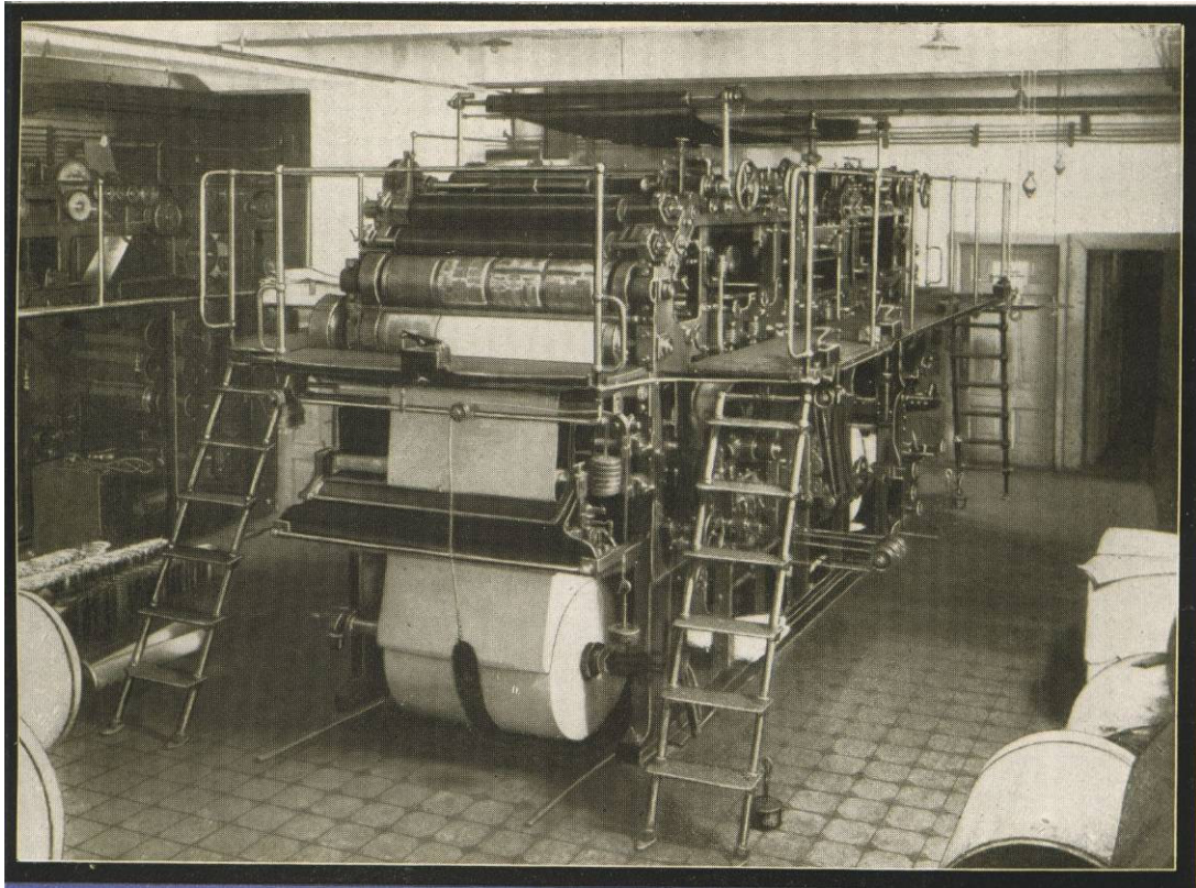
RÉSZLET A ROTÁCIÓS GÉPTEREMBŐL
