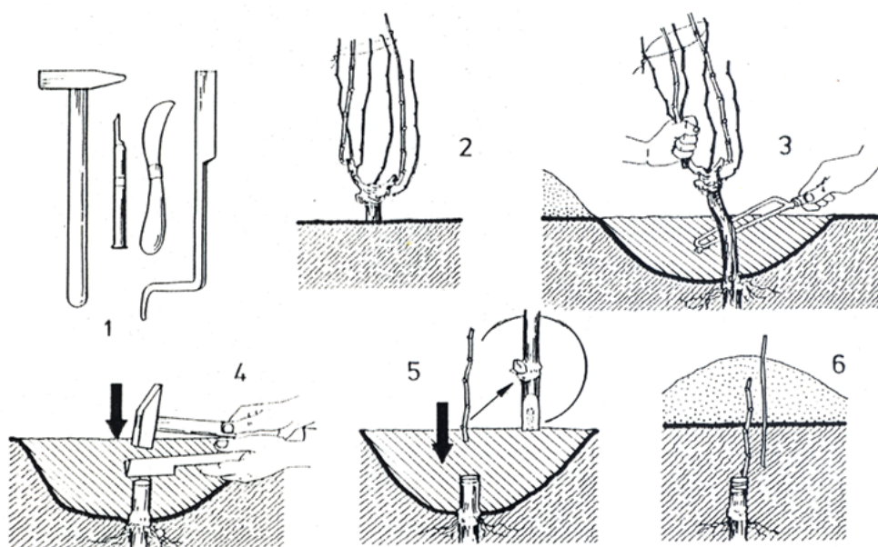
53. ábra. A gyökértörzsbe oltás 1) az oltás eszközei; 2) az alanytőke; 3) az oltási helyen a gyökértörzs elfűrészelése; 4) hasítékvágás az alanyon; 5) az oltócsap elkészítése; 6) a kész oltvány (Kozma, 1991)
