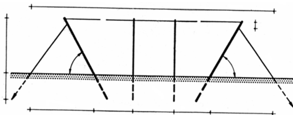
70. ábra. Az egyesfüggöny-műveléshez alkalmas támrendszer A MI-08-0003-83 sz. műszaki irányelvek által ajánlott támberendezés vázlata
