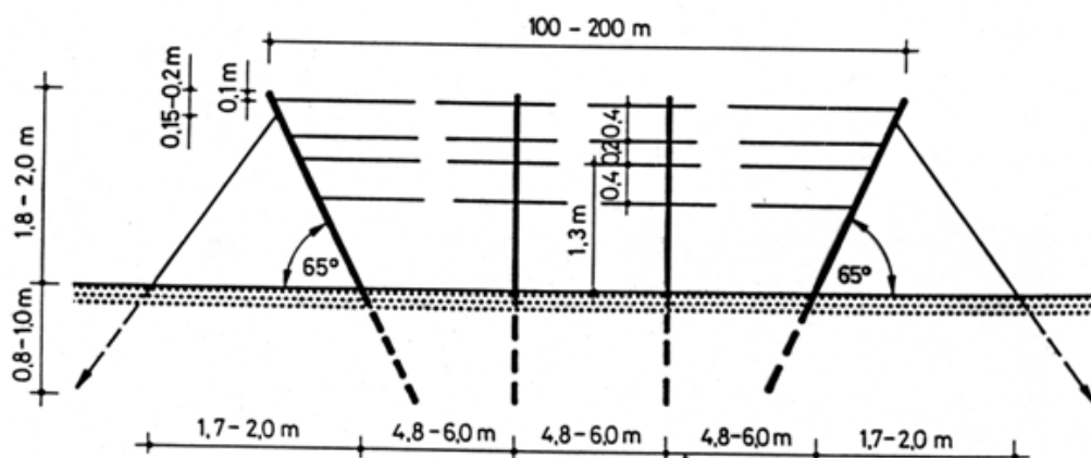
69. ábra. A MI 08-0003-83 sz. műszaki irányelvek által ajánlott támberendezés magas kordon- (Moser-, Sylvoz, ernyő) műveléséhez
