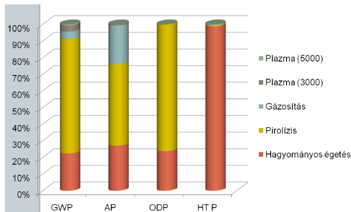
13. ábra Egyes környezeti mutatók százalékos értéke különféle termikus technológiáknál
