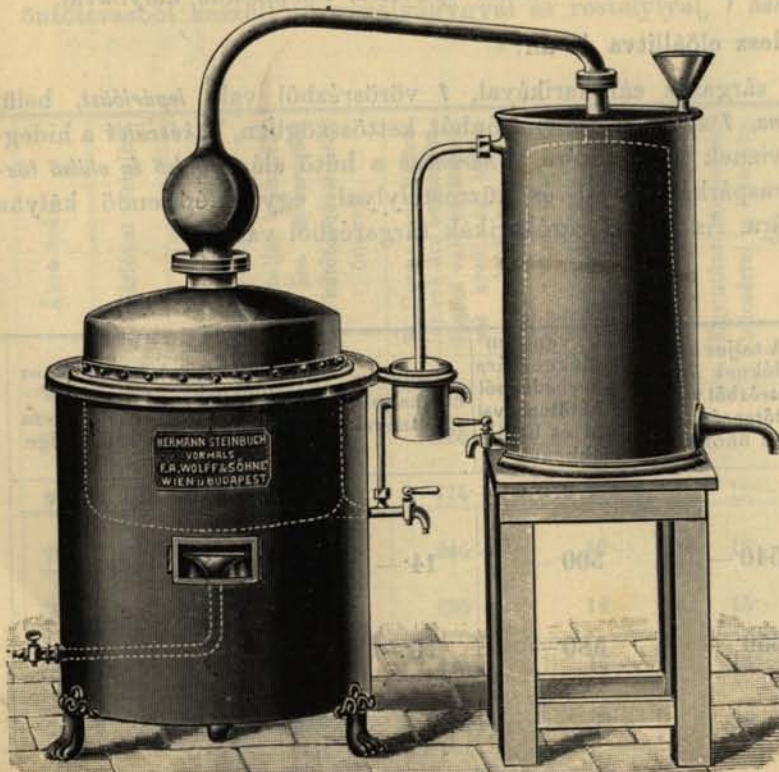
Ábra 711. Vízleparlókészülék, újabb szerkezetű, a 710. ábra alattiaknak megfelelően, de légszesztüzelésre berendezve, megfelelő, jó csappal ellátott gázégővel és kovácsoltvas kályhával.
