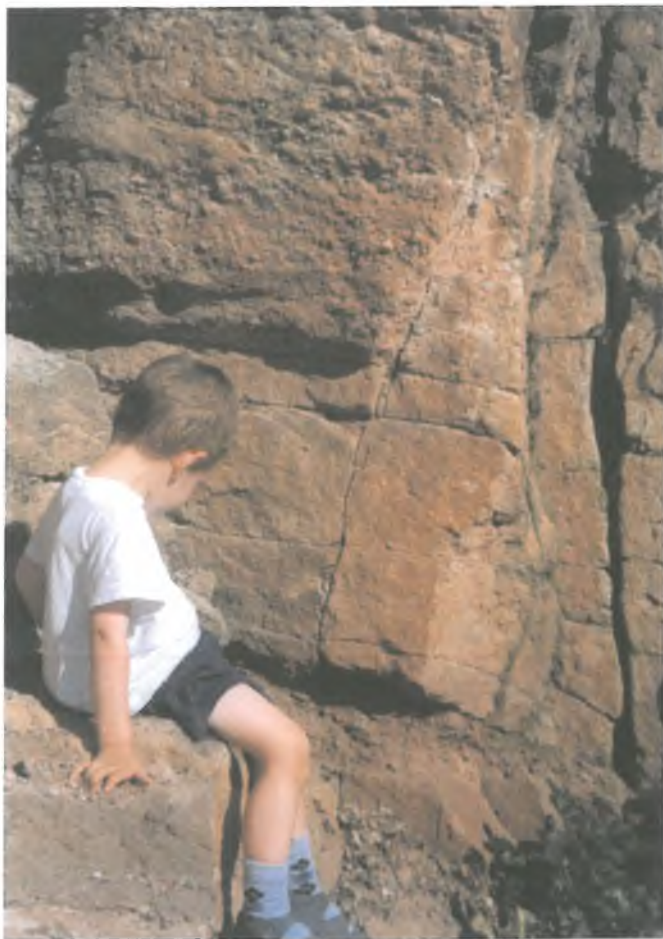
Vegyes szemnagyságú felső-permi homokkő Káptalanfüreden, a Kőcsi-tó melletti hajdani (védett) kőbányában
