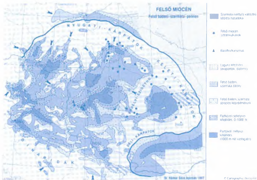
A Kárpát-medence ősföldrajzi képe a miocén végén (Szerk.: Hámor G., megjelent: Magyarország atlasza, Cartographia)
