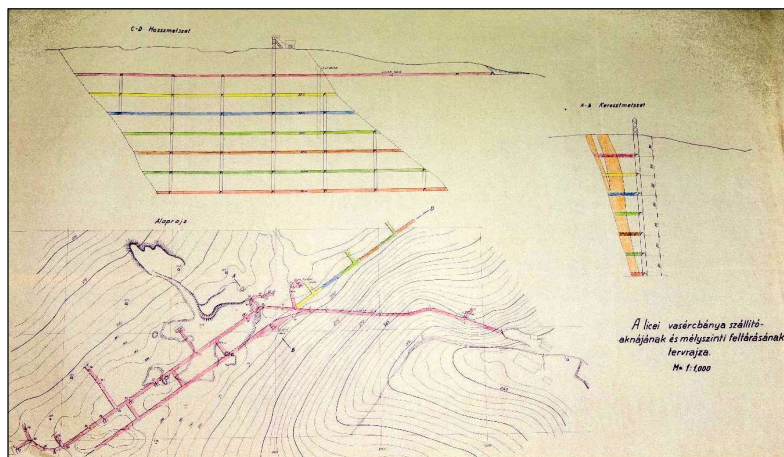
A licei bánya szállítóaknájának és további feltárásának a tervrajza. 111 (Fotó: Breznánik Peter.)
