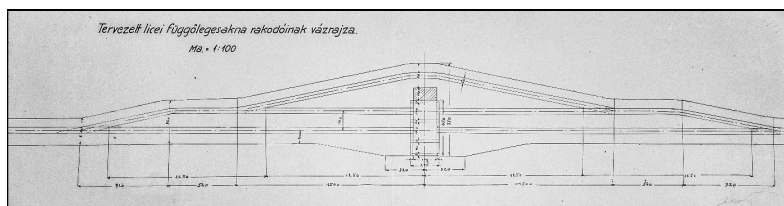
A tervezett függőakna rakodóinak tervrajza. 112 (Fotó: Breznánik Peter.)
