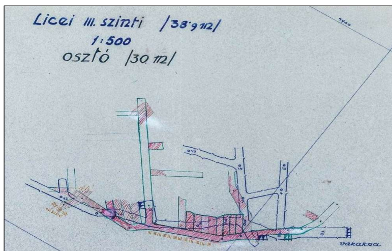
A 30-as osztószint térképe. 110 (Fotó: Breznánik Peter.)
