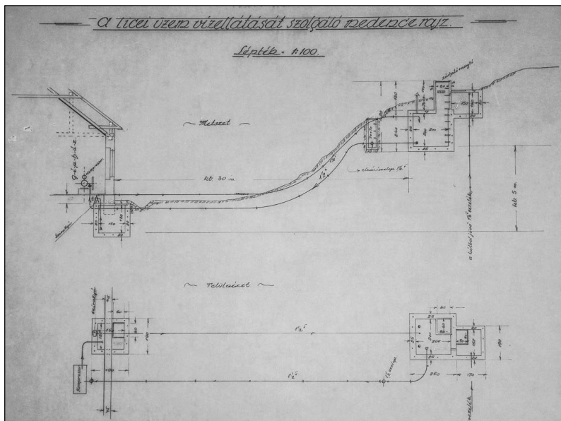
Az üzem vízellátását szolgáló medence vázlata. 103 (Fotó: Breznaník Peter.)
