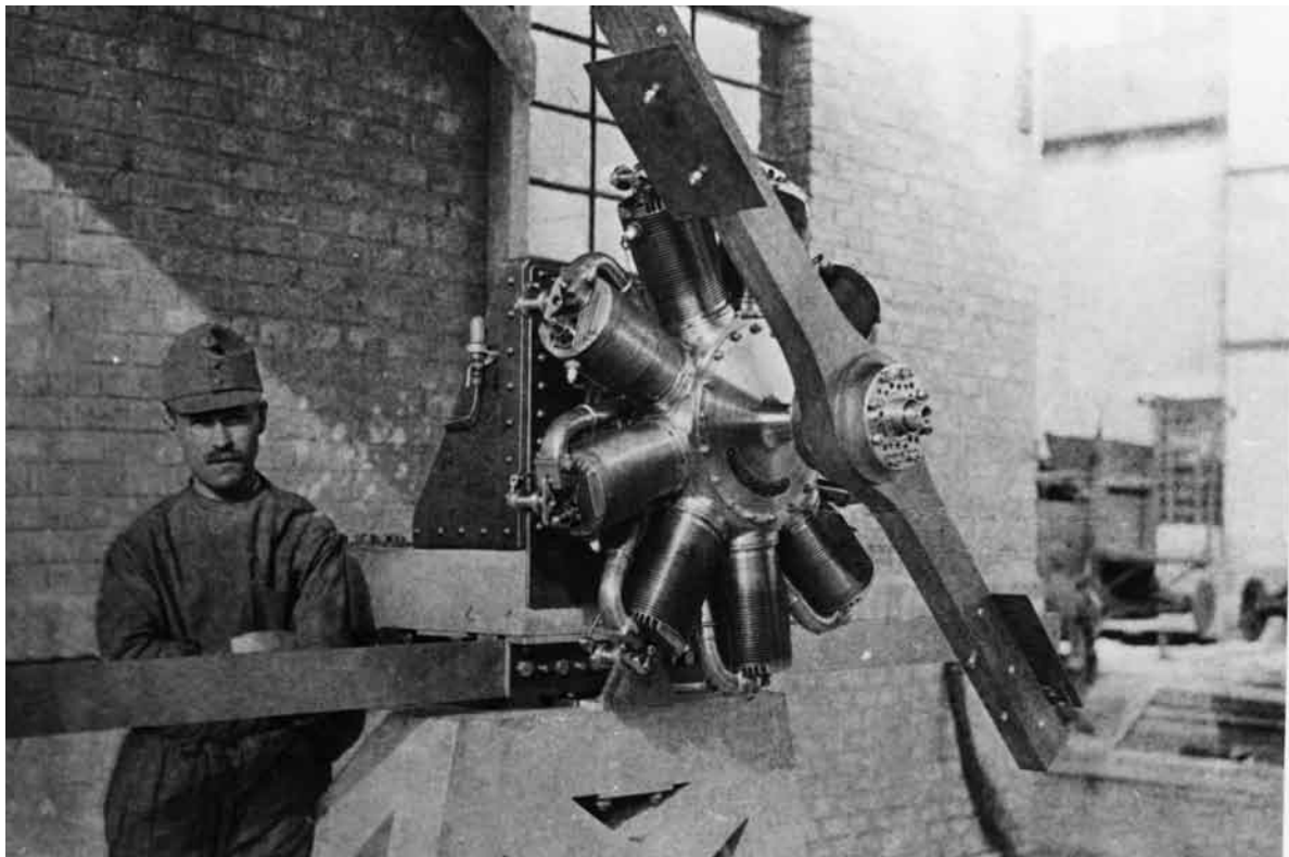
Pestszentlőrinci helikopterkísérletek: helikopter megfigyelőkosárral (fent); helikoptermotor a próbapadon (lent)
