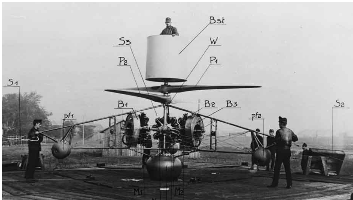
Pestszentlőrinci helikopterkísérletek: helikopter megfigyelőkosárral (fent); helikoptermotor a próbapadon (lent)
