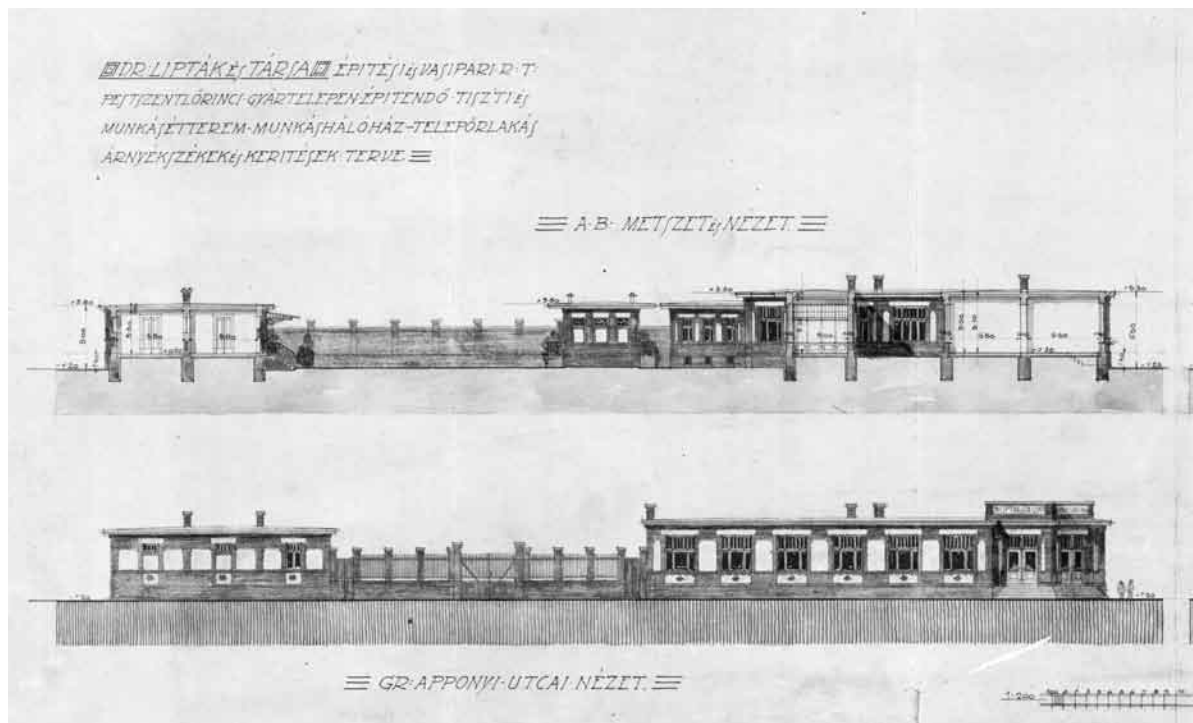
Lipták-gyári étkező és hálókáz, tervrajz, 1916
