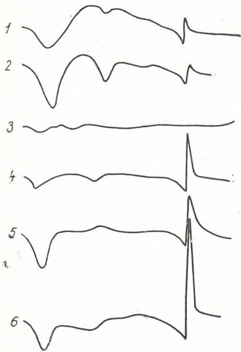
29. ábra. Szepiolit DTA-görbéi
