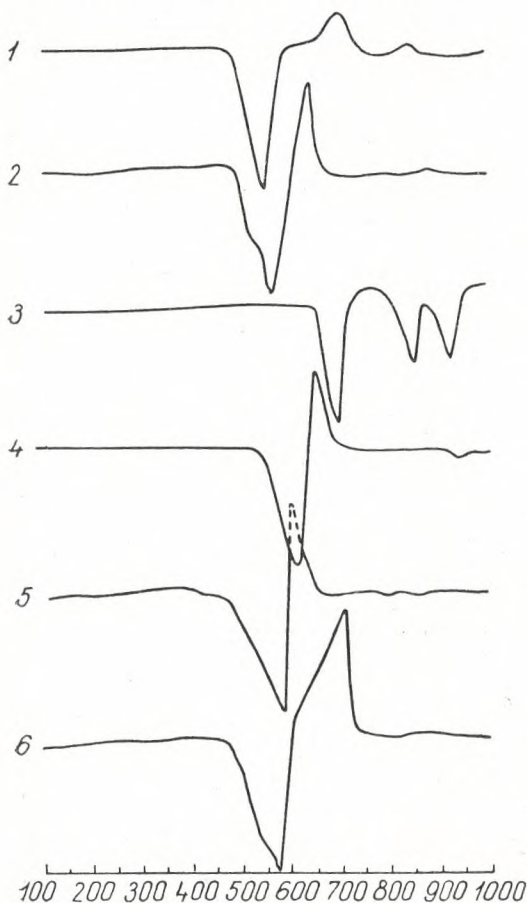
56. ábra. Karbonátok DTA-görbéi
