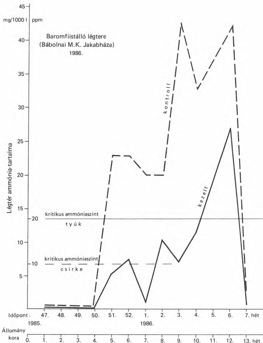
15. ábra. Az ammónia-tartalom változása alginites kezelés hatására mélyalmos baromfiistálló légtérében (SZABÓ V. és FEKECS L. vizsgálataira alapján)
