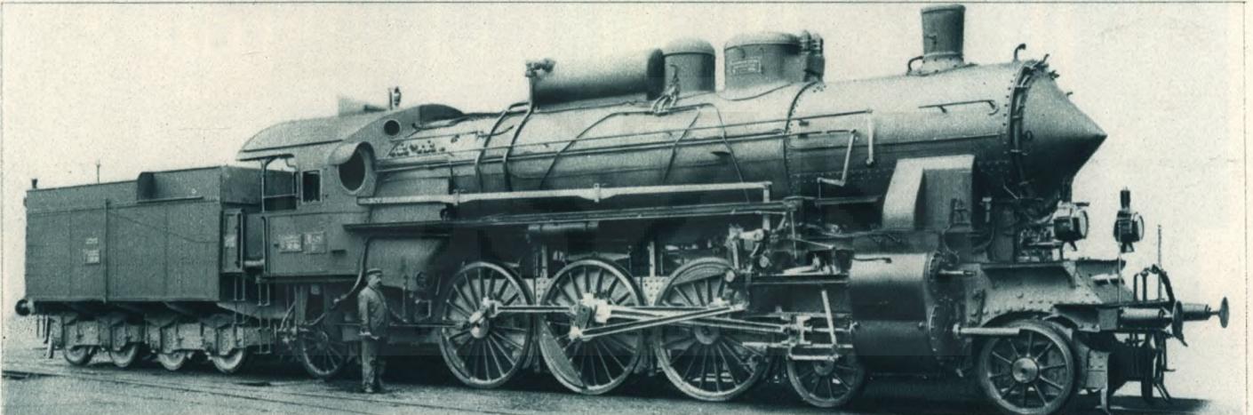
Magyar Királyi Államvasutak 301. sorozatú mozdonya. Nehéz személy- és gyorsvonatokhoz. — Die Lokomotive der k. u. Staatsbahnen Serie 301. Zu schweren Personen- und Eilzügen. — Locomotive des Chemin de Fer Roy. Hongrois, de la série 301. Pour trains rapides et convois lourds de trains omnibus. — The locomotive 301 series of the Royal Hungarian State Railways. For heavy passenger and fast trains.
