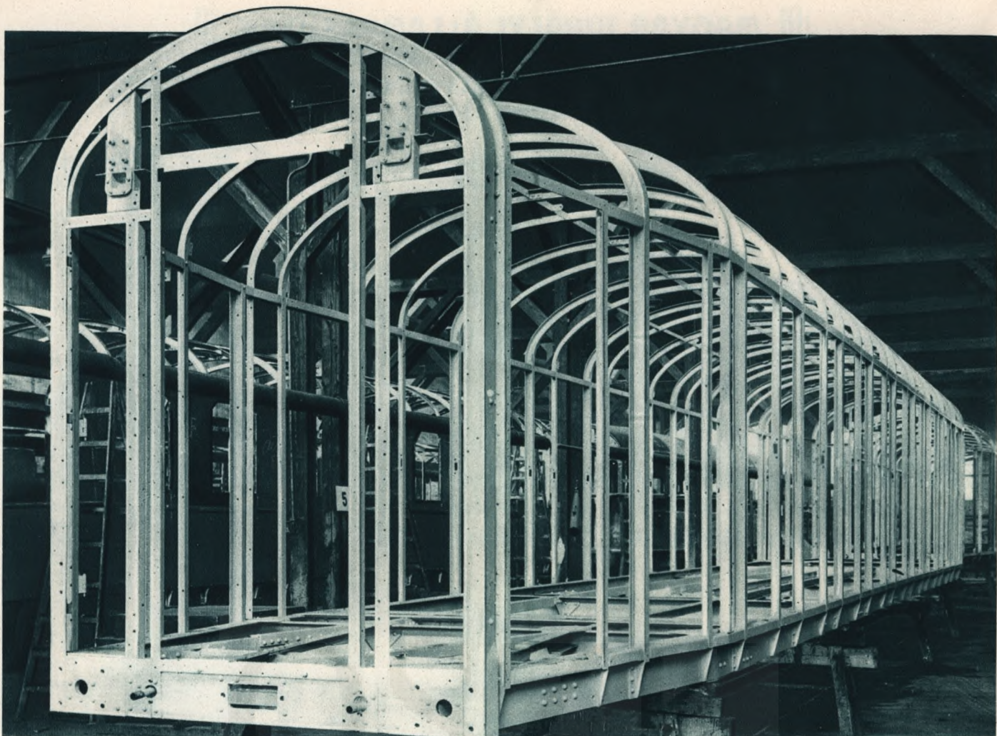
Vasvázis négytengelyű III. osztályú kocsik szkevényváza. Új kocsik, nemzetközi gyorsvonatok részére. — Kastengerippe zu Wagen III. Klasse mit Eisengerippe und 4 Achsen. Neue Wagen zu internationalen Eilzügen. — Cadre de carrosserie d'un wagon de IIIe classe à quatre essieux armature de fer. Voitures neuves pour trains internationaux. — Boot-frame-work of a III. Class-waggon with iron-frame and four axles. New waggons for international express trains.
