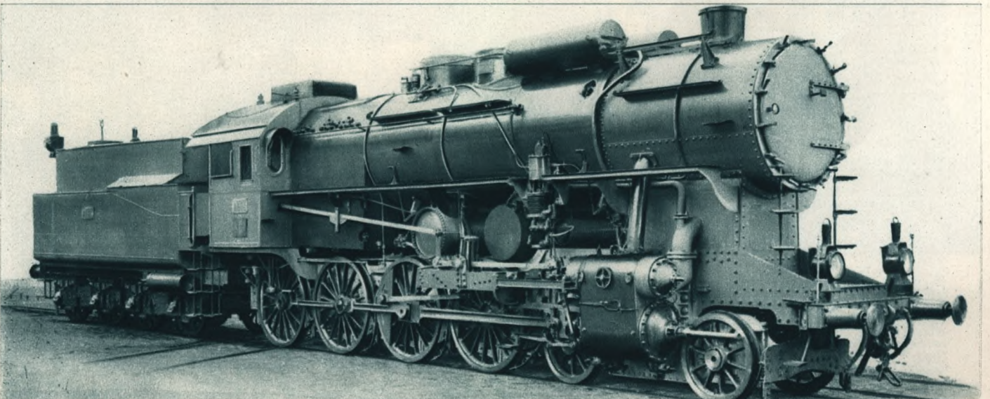
Magyar Királyi Államvasutak 424. sorozatú mozdonya. Nehéz személy- és gyorsvonatokhoz. — Die Lokomotive der k. u. Staatsbahnen Serie 424. Zu schweren Personen- und Eilzügen. — Locomotive Chemin de Fer Roy. Hongrois, de la série 424. Pour trains rapides et convois lourds de trains omnibus. — The locomotive 424. series of the Royal Hungarian State Railways. For heavy passenger and fast trains.
