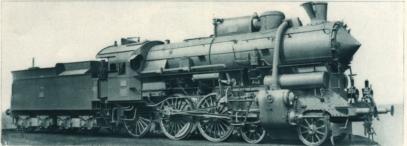
Magyar Királyi Államvasutak 328. sorozatú mozdonya. Nehéz személy- és gyorsvonatokhoz. — Die Lokomotive der kön. ung. Staatsbahnen Serie 328. Zu schweren Personen- und Eilzügen. — Locomotive des Chemin de Fer Roy. Hongrois, de la série 328. Pour trains rapides et convois lourds de trains omnibus. — The locomotive 328. series of the Royal Hungarian State Railways. For heavy passenger and fast trains.
